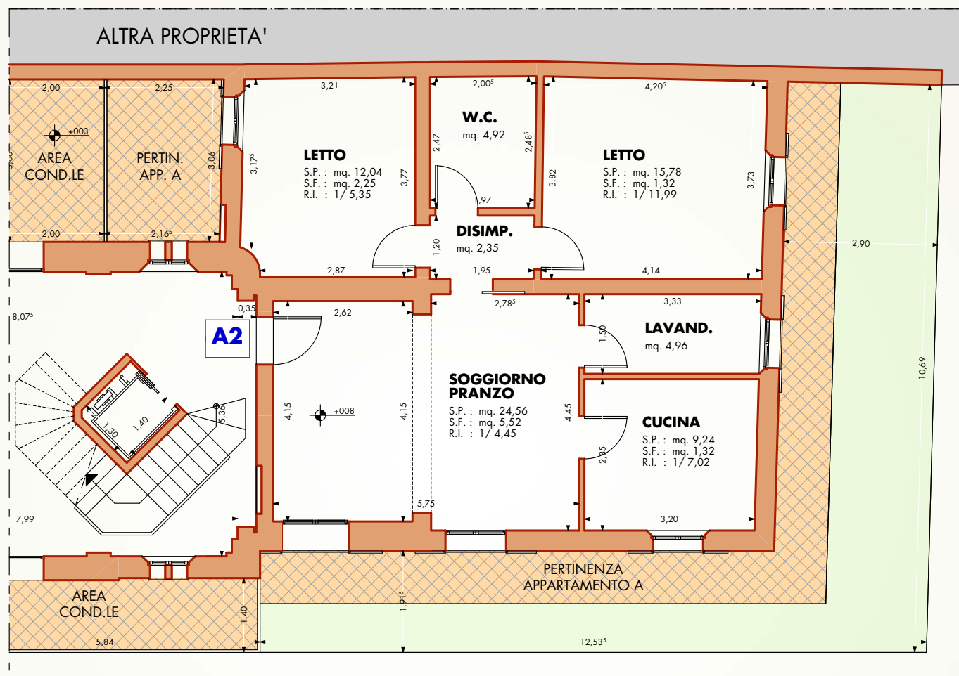
PLANIMETRIA TECNICA
