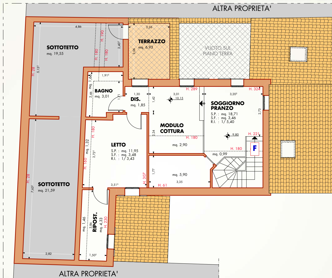
PLANIMETRIA TECNICA
